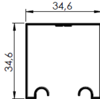
601040009 - PESO 0,334 kg/m 8 BARRAS POR PACOTE
