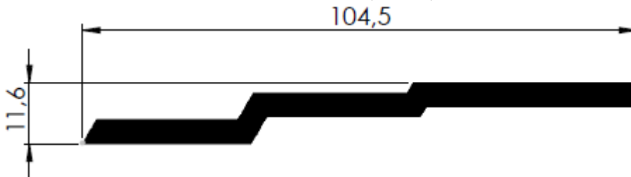
601200008 - PESO 1,400 kg/m 3 BARRAS POR PACOTE
