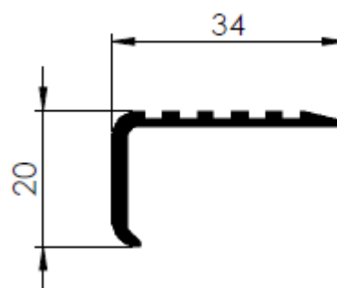
CANTO DE ESCADA
