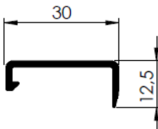
601130016 - PESO 0,273 kg/m 20 BARRAS POR PACOTE
