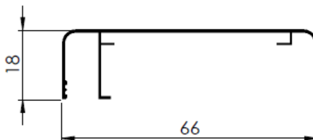
LATERAL GRANDE
