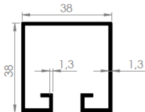
2 ROLDANAS RETAS
