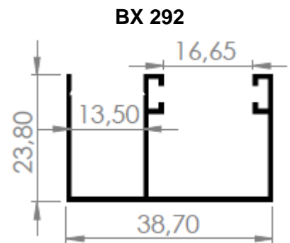
BX 292 601120010 - PESO 0,335kg/m 10 BARRAS POR PACOTE
