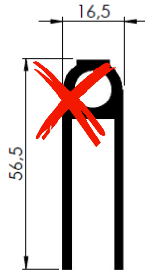
TRINCO 56,5 X 16,5MM
