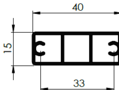
601070010 - PESO 0,545 kg/m 8 BARRAS POR PACOTE
