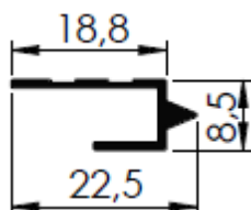
CASE 05 22,5 X18,8MM
