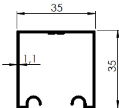
601040001 - PESO 0,388kg/m 8 BARRAS POR PACOTE
