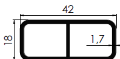
601070011 - PESO 0,579 kg/m 10 BARRAS POR PACOTE
