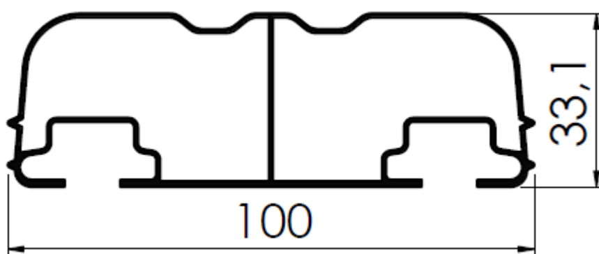
601270008 - PESO 0,943 kg/m- 3 BARRAS POR PACOTE
