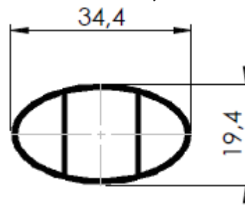
601110006 - PESO 0,388 kg/m 10 BARRAS POR PACOTE
