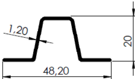
TRAPÉZIO LEVE
