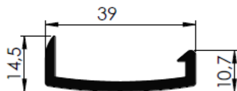
601130086 - PESO 0,409 kg/m 10 BARRAS POR PACOTE
