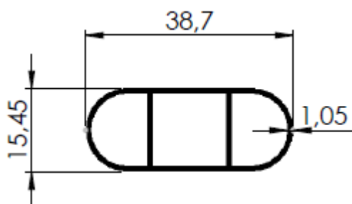
OBLONGO 38,7 x 15,5 x 1,05MM
