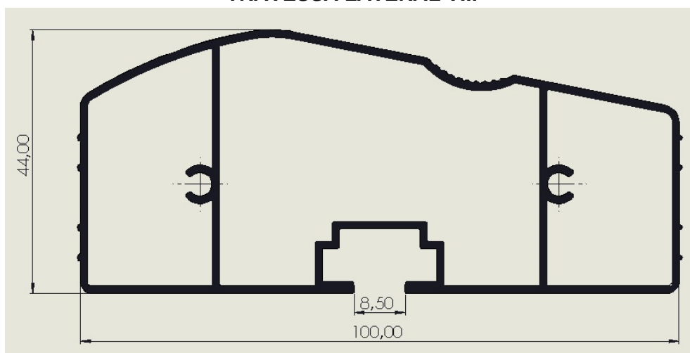
601270028 - PESO 1,195 kg/m- 3 BARRAS POR PACOTE
