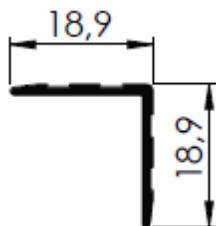
CASE 03 18,9 X18,9MM
