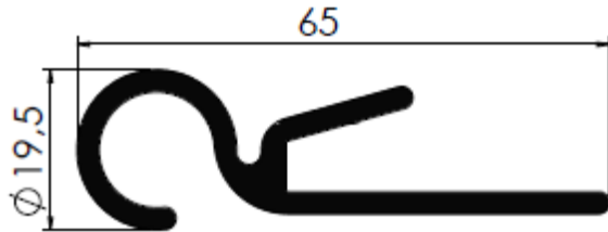
ESTICADOR DE LONA SIDER MODELO FC
