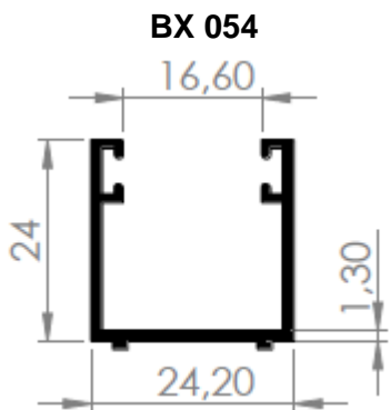
BX 054 601120014 - PESO 0,308kg/m 10 BARRAS POR PACOTE
