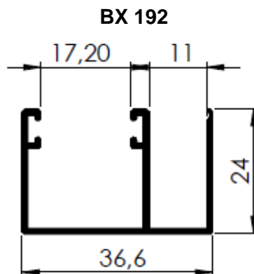
BX 192 601124882 - PESO 0,368kg/m 10 BARRAS POR PACOTE
