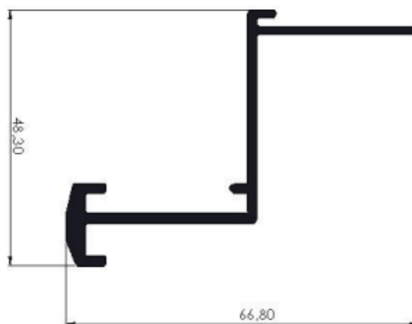
CONTORNO DE PORTA GRANDE 66,80 X 48,3 X 35,2MM
