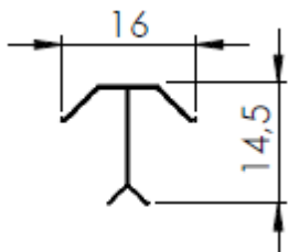
CANTONEIRA SEXTAVADA ALTA
