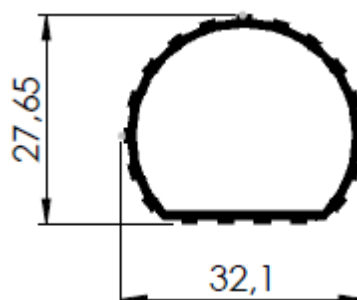
601130023 - PESO 0,376 kg/m - 10 BARRAS POR PACOTE
