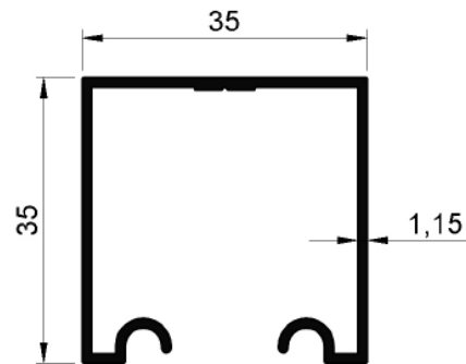
2 ROLDANAS CONCAVAS
