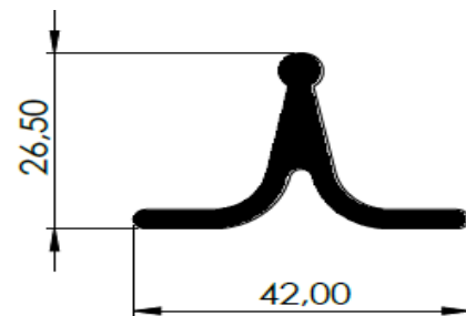
QUILHA
