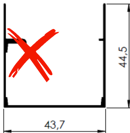
TRILHO SUP. BOX LISO 43,7MMX44,5MM
