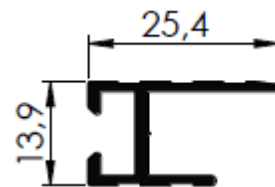
CASE 02 25,4 X13,9MM
