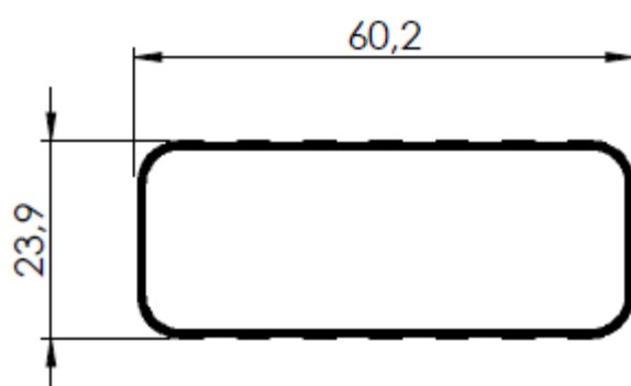
601130024 - PESO 0,541 kg/m - 10 BARRAS POR PACOTE
