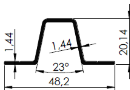
TRAPÉZIO 4
