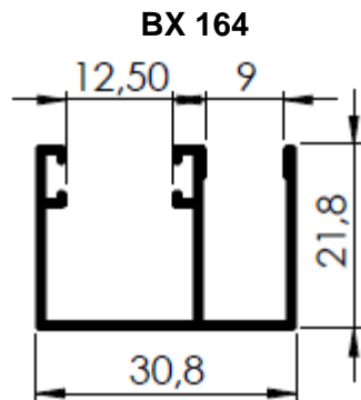
BX 164 601122015 - PESO 0,318kg/m 10 BARRAS POR PACOTE
