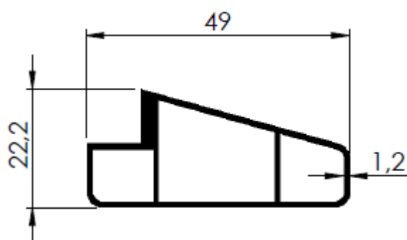
601080001 - PESO 0,546 kg/m 10 BARRAS POR PACOTE
