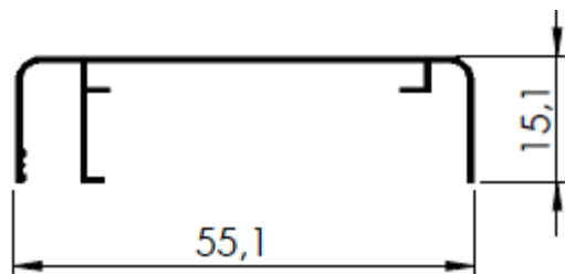
LATERAL PEQUENA
