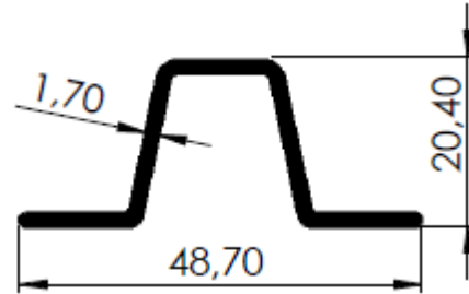
TRAPÉZIO NORMAL
