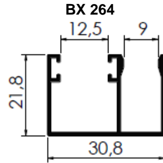
BX 264 601120018 - PESO 0,293 kg/m 10 BARRAS POR PACOTE
