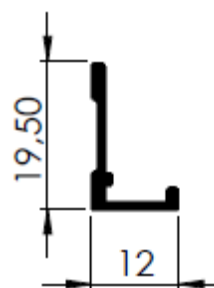
1 ROLDANA RETA
