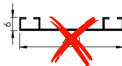
TRILHO INFERIOR 47,1 X 5,7 X 0,7MM
