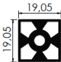
601140027 - PESO 0,558 kg/m 8 BARRAS POR PACOTE
