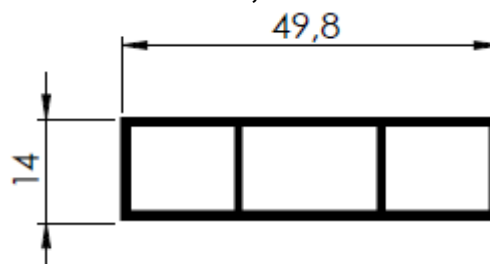
TRAVESSA 49,8 X 14 X 1,2MM
