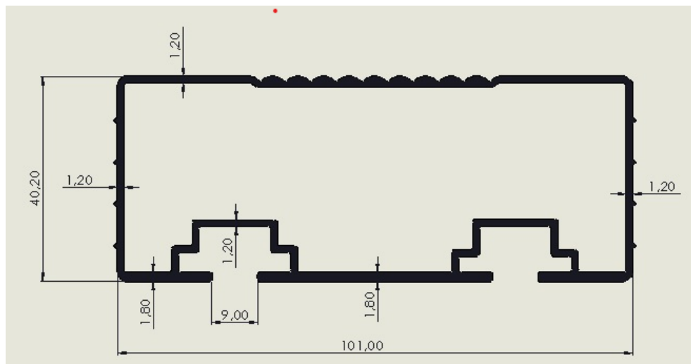
601270027 - PESO 1,273 kg/m- 3 BARRAS POR PACOTE
