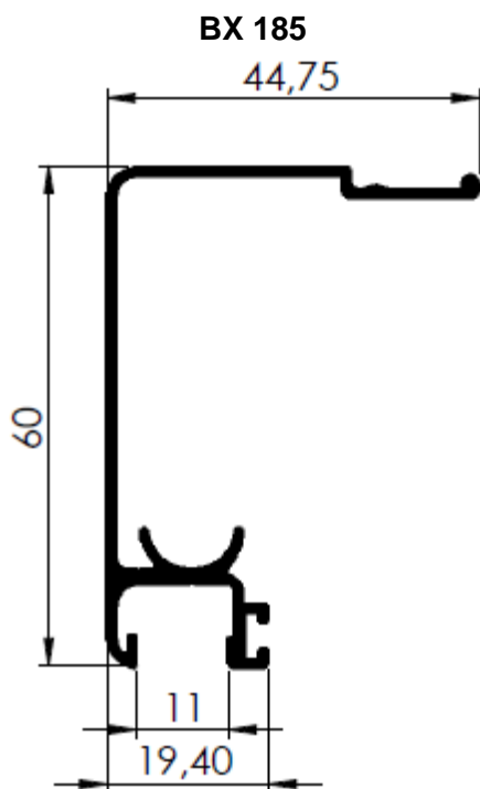
601125012 - PESO 0,514kg/m 10 BARRAS POR PACOTE
