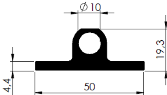
FECHO FEMEA50,0x4,4MM
