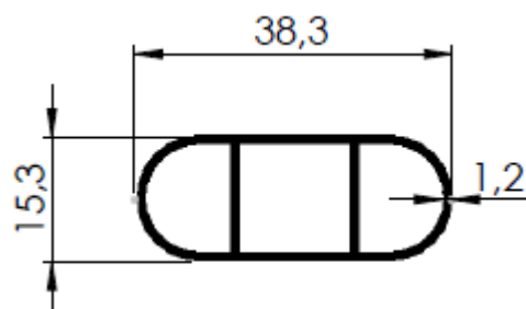
OBLONGO 38,7 x 15,5 x 1,2MM
