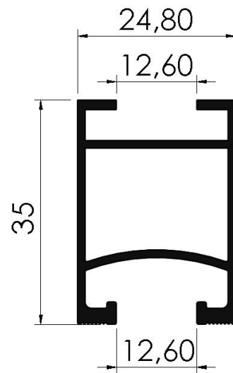
601260024 - PESO 0,510 kg/m 8 BARRAS POR PACOTE
