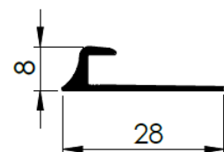
PERFIL "J" BAÚ III (PINGADEIRA)
