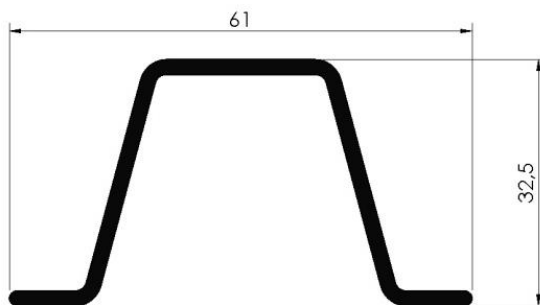
TRAPÉZIO 61 X 32,5
