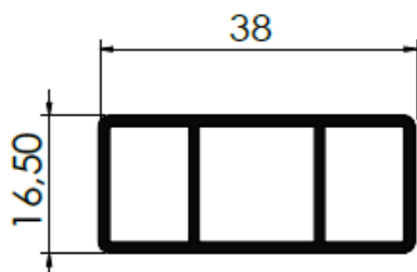
601070015 - PESO 0,473 kg/m 10 BARRAS POR PACOTE
