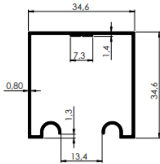
601040011 - PESO 0,315kg/m 8 BARRAS POR PACOTE
