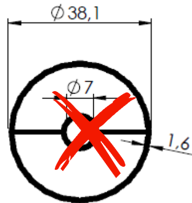
601140004 - PESO 0,735 kg/m 6 BARRAS POR PACOTE
