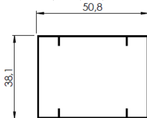
601070015 - PESO 0,530 kg/m
