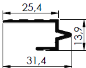
CASE 01 31,4 X13,9MM
