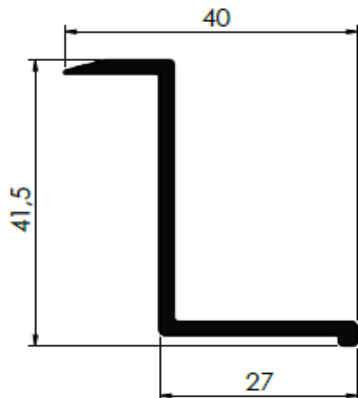
601260017 - PESO 0,441 kg/m 12 BARRAS POR PACOTE
