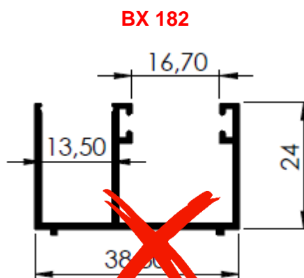
BX 182 601125017 - PESO 0,410kg/m 10 BARRAS POR PACOTE
