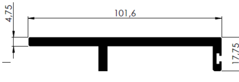
PERFIL "F" DESLIZANTE
