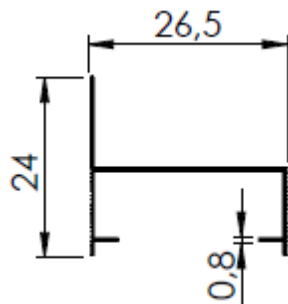
CONTRA MARCO
