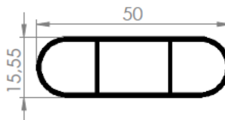
OBLONGO 49,8 x 15 x 1,15MM
