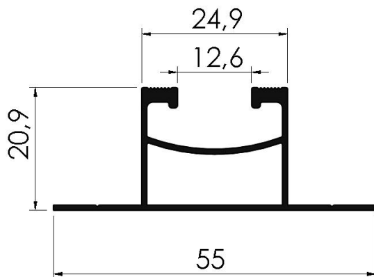
601260023 - PESO 0,383 kg/m 10 BARRAS POR PACOTE
