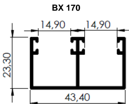
BX 170 601124751 - PESO 0,475kg/m 10 BARRAS POR PACOTE
