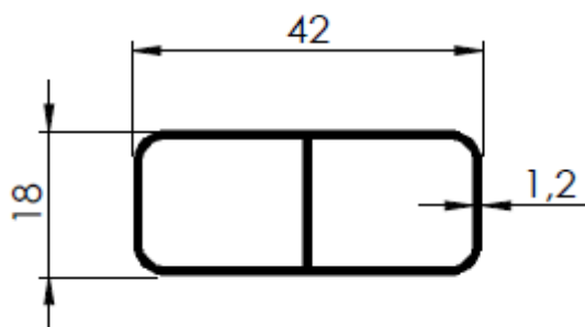
601071592 - PESO 0,415 kg/m 10 BARRAS POR PACOTE
