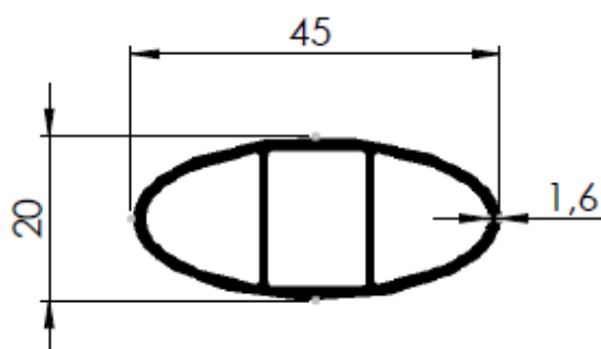
601110005 PESO 0,544 kg/m 10 BARRAS POR PACOTE
